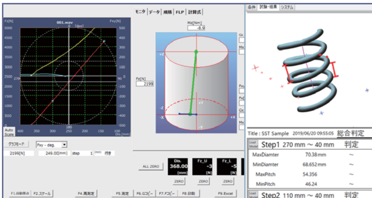
4台のレーザーによる外径測定イメージ
