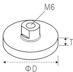
平型圧子 ステンレス製 CT-F[D]
