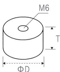
平型圧子 ジュラコン製 CJ-F[D]-T
